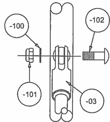
DETAIL B-B (TYP. OF 2 PL.)
